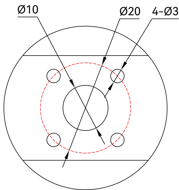
局部视图 比例2:1
