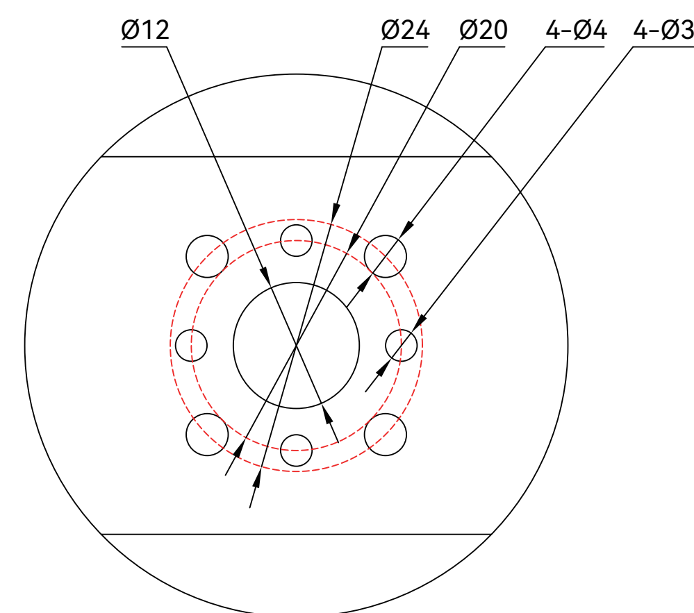
局部视图 比例2:1
