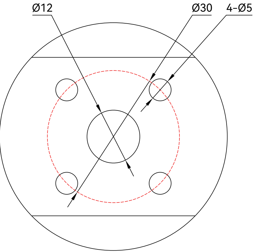
局部视图 比例2:1
