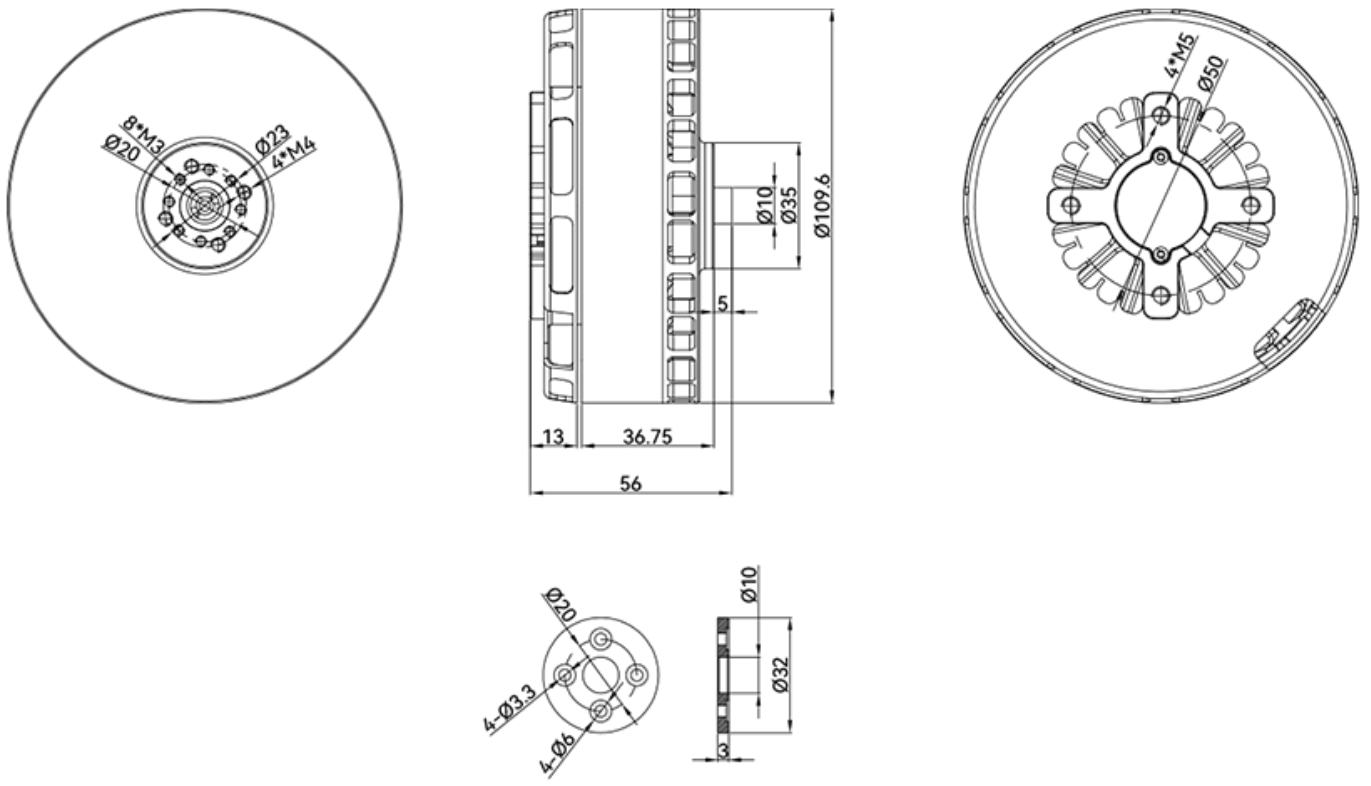
【电机】
