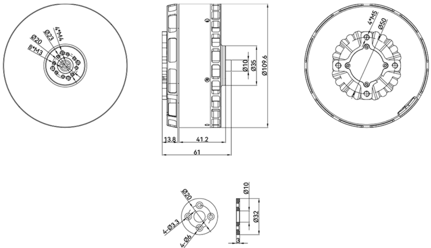
【电机】
