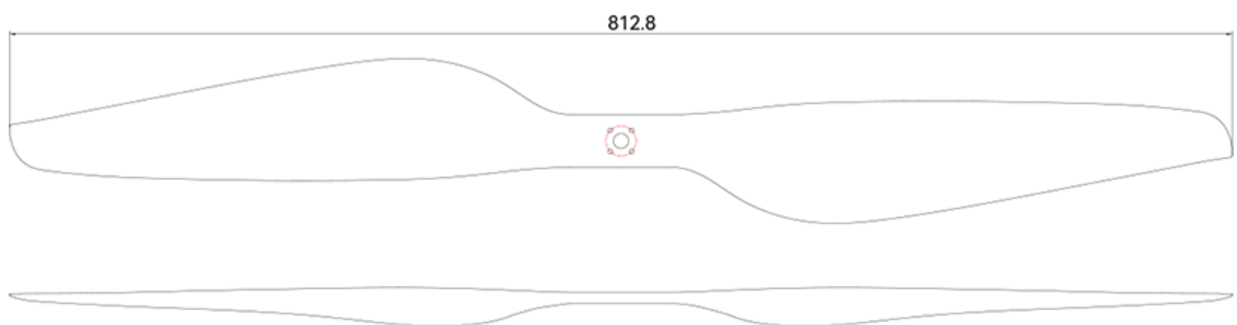
【桨】
