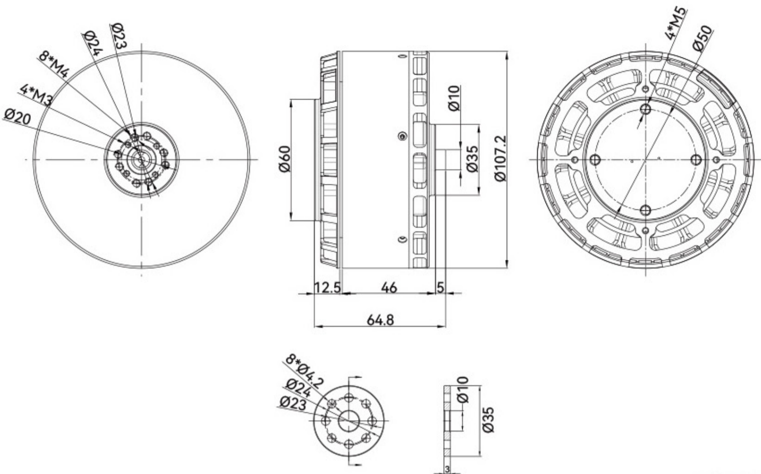
【MOTOR】
