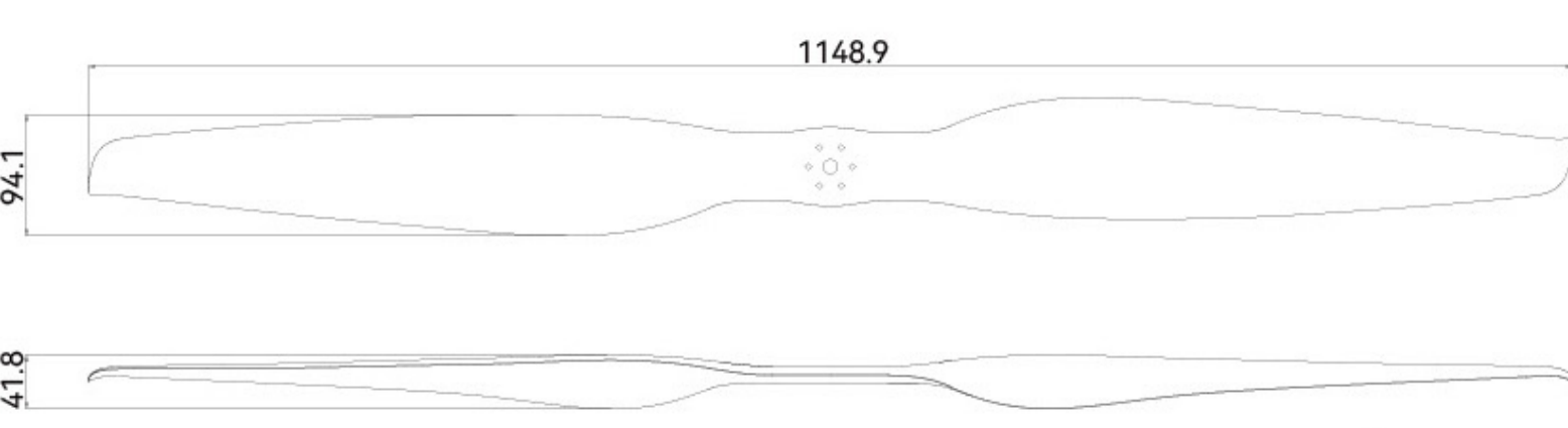
【PROPELLER】
