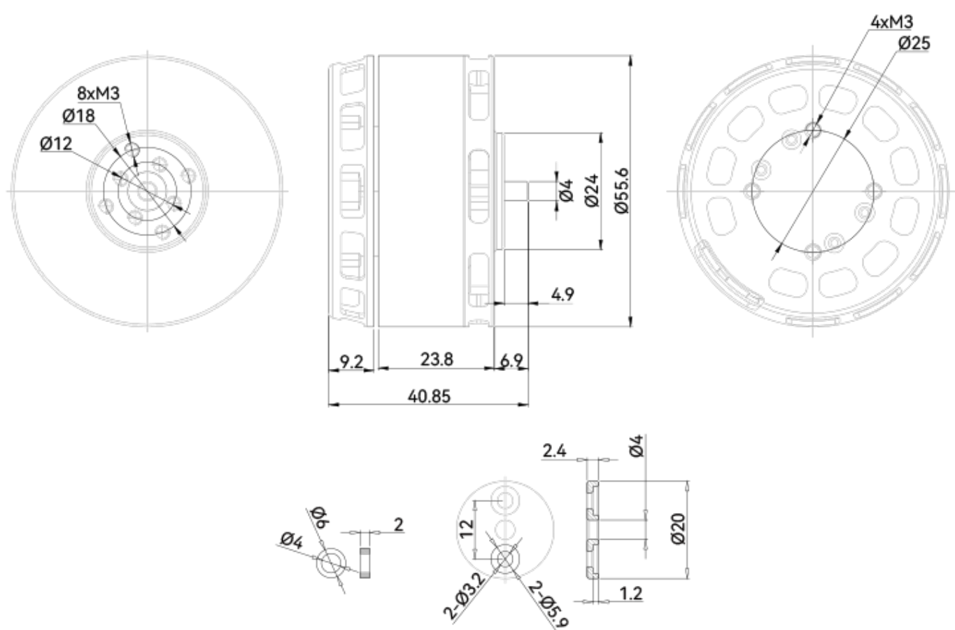
【电机】
