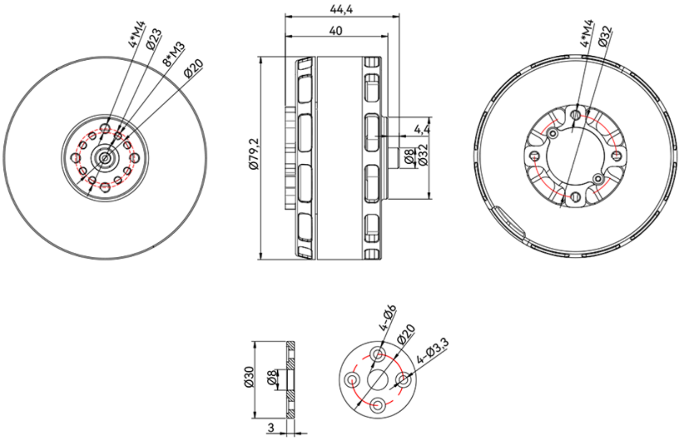
[MOTOR]
