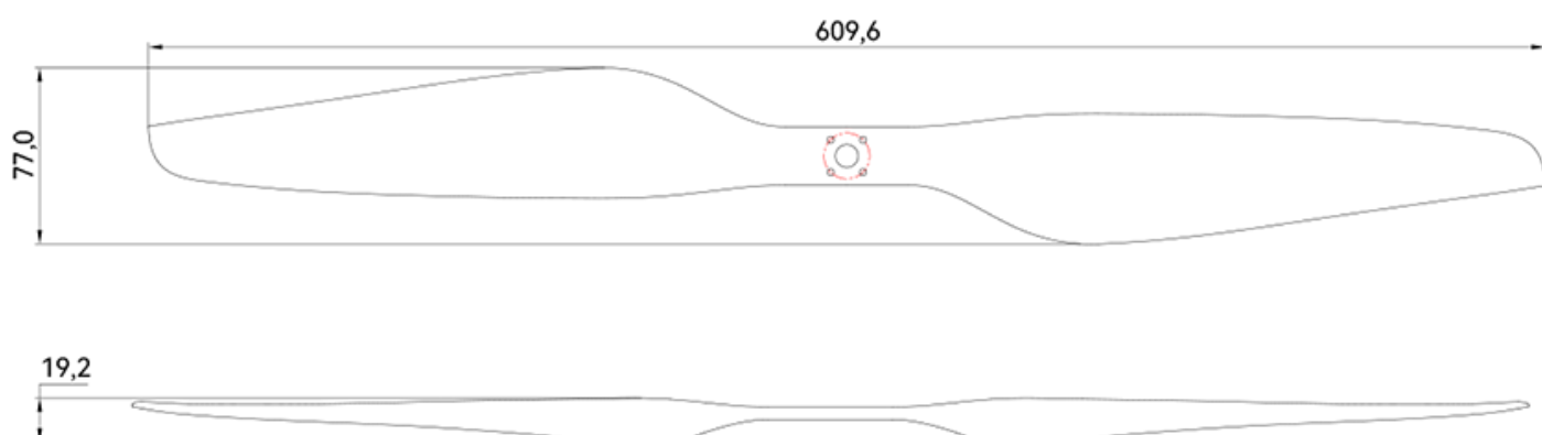
【桨】
