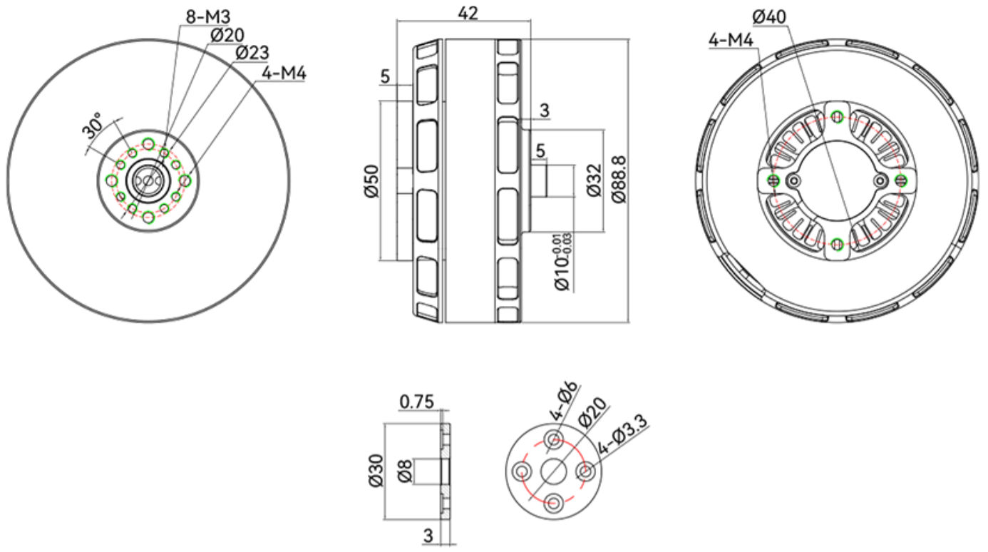
【MOTOR】
