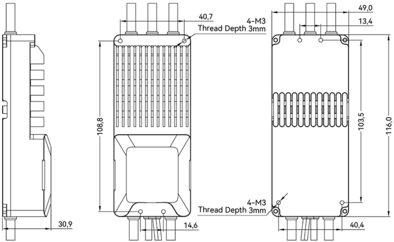
【ESC】
