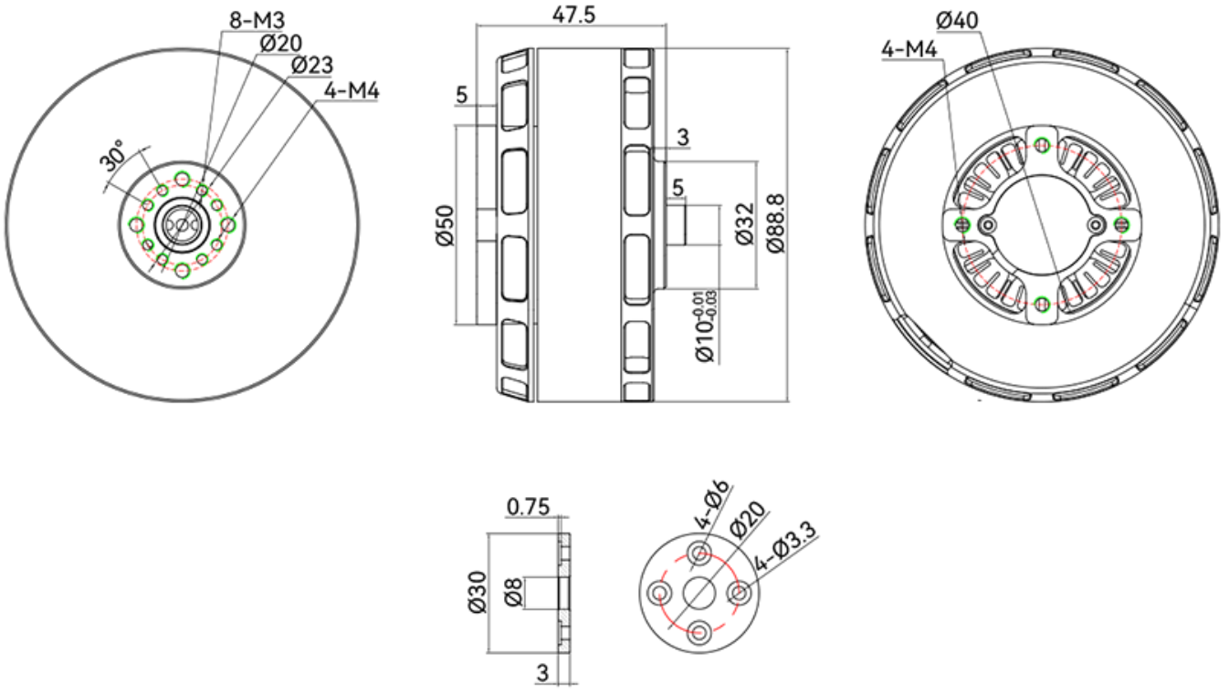
【MOTOR】
