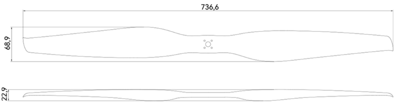
【PROPELLER】
