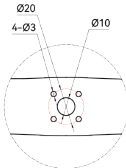
局部视图 比例2:1
