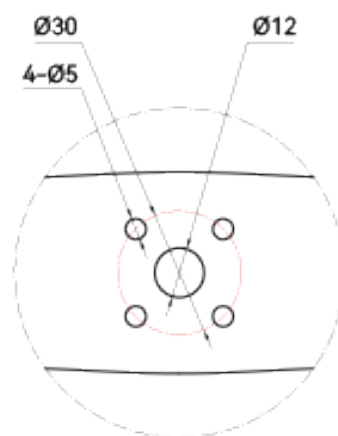
局部视图 比例2:1
