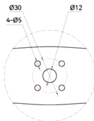
局部视图 比例2:1
